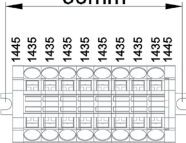
TIP-2 SET (MAVI) 53mm
